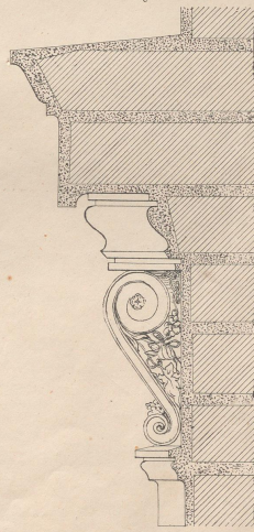
Fensterüberdachung mit Consolen.
