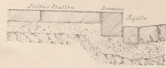
Reguläres Plattenpflaster. Profil.
