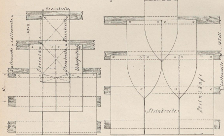
Eindeckung nach deutscher Methode auf Brettverschallung. Ansicht.
