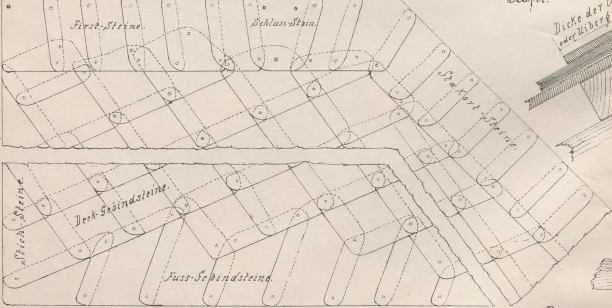
Detail in halber Naturgrösse für die doppelte Eindeckung. Schnitt.
