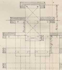
Detail der Überbindung in halber Naturgrösse. Schnitt.
