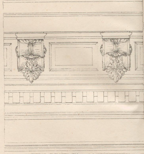
mit Consolen. Ansicht.
