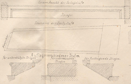
Detaile der Stufen
