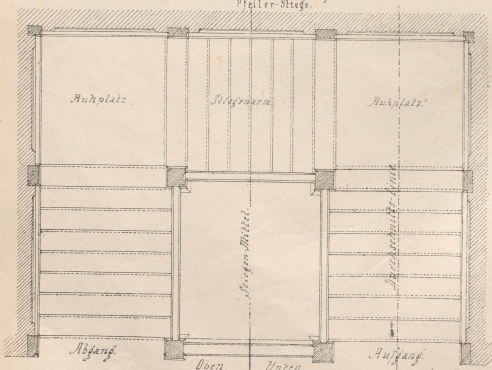
Grundriss der dreistufigen geraden Pfeiler-Stiege
