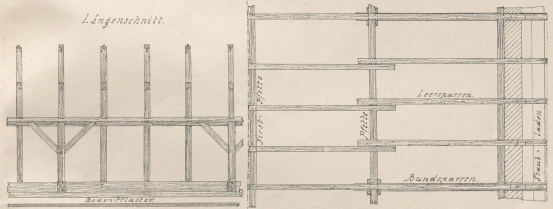
Grundriss.
