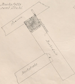
Pfettenauflager auf Kränzen.
