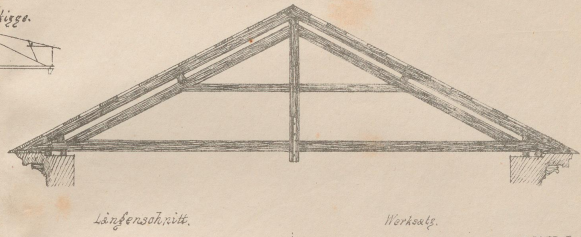
Hängwerk mit zusammengefügtter Hängsäule.
