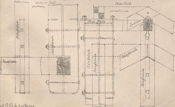
Detail der doppelten Hängsäule.
