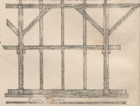
Detail der einfachen Hängsäule.
