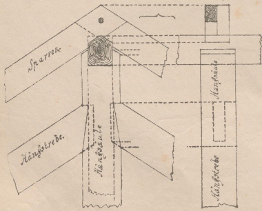
Detail der einfachen Hängsäule.
