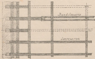
Detail der einfachen Hängsäule.
