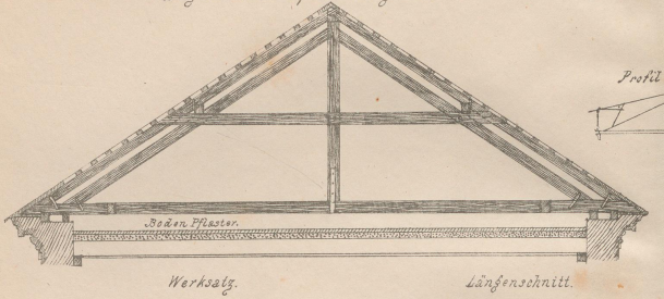
Hängwerk mit einfacher Hängsäule.
