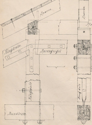
Detail des Häng- u. Sprengwerkes.
