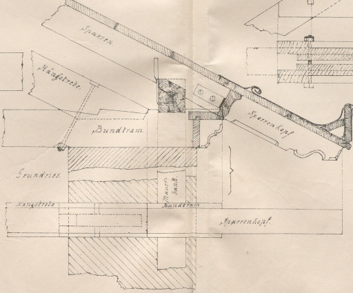
Detail des Sparrenkopfes.
