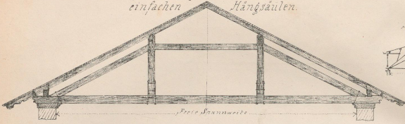
Längenschnitt.
