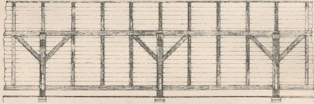
Detail des Häng- u. Sprengwerkes.
