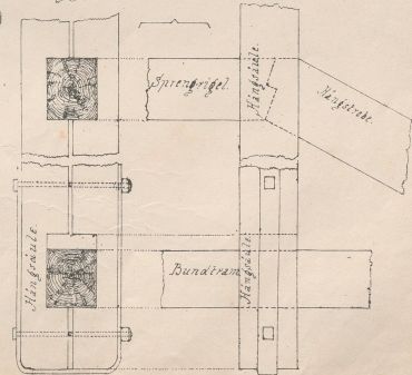
Detail des Sprengwerkes.
