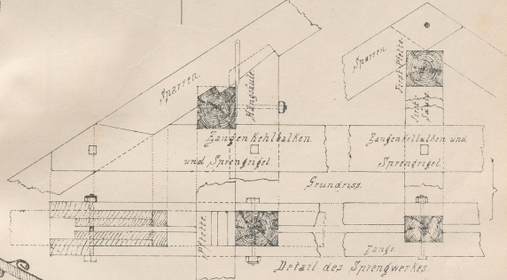
Detail des Hängwerkes.
