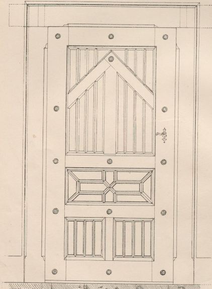
Detail der Hausthüre in halber Naturgröße
