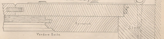
Detail des Flügels in halber Naturgröße
