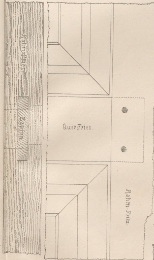
Fries Verzäpfung in halber Naturgröße.
