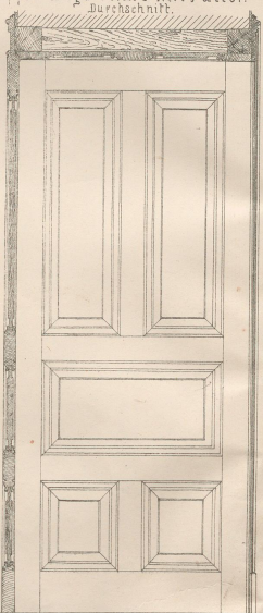
Fünffüllungs Thür mit Futter.
