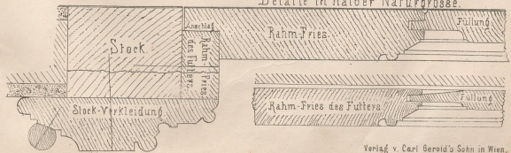
Details in halber Naturgröße.
