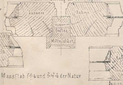
Mittelanschlag der Oberflügel.
