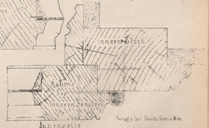
Seitenanschlag in Naturgrösse.
