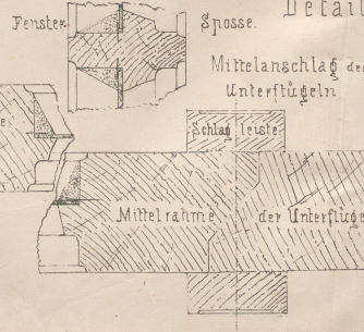
Details in Naturgrösse.
