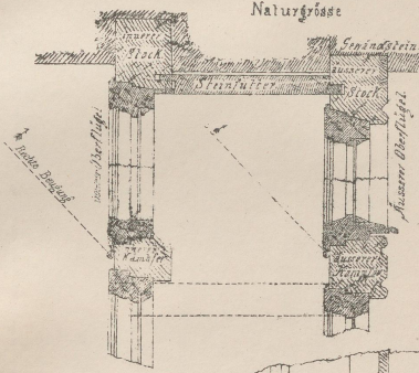
Profil in \frac{1}{2} der Naturgröße
