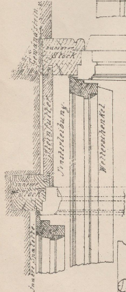
Grundrisse des Fensters.
