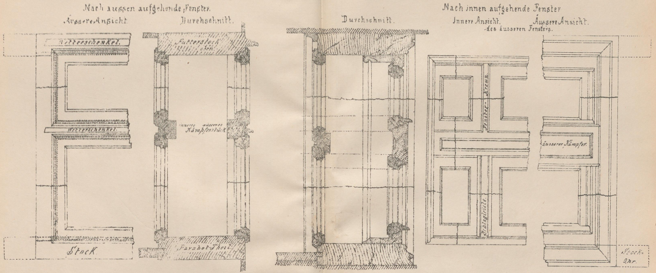
Grundrisse der Futterstöcke
