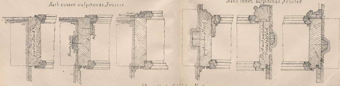
Grundrisse der Futterstöcke
