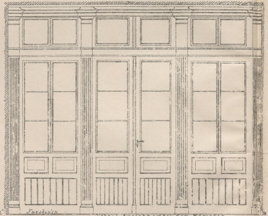
Abschlusswand mit Glashüren und Fenstern Ansiicht.
