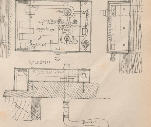
Überbautes Riegelschloss mit schliessender Falle
