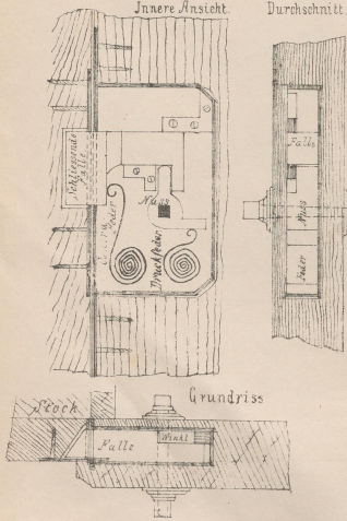
Ein festemtes Fallenschloss
