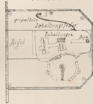
Grundriss.
