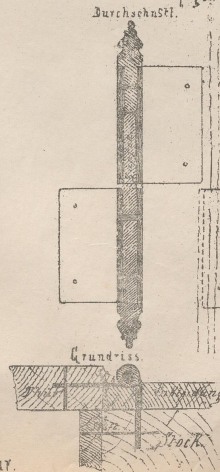
Aufsatzbänder [gewöhnliche]
