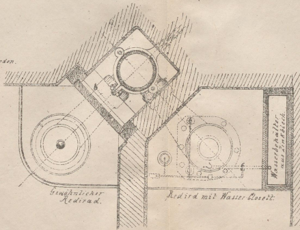
Grundriss oberden Sitzbrettern.
