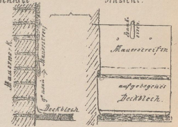
Eindeckung der Mauerviren Durchschnit
