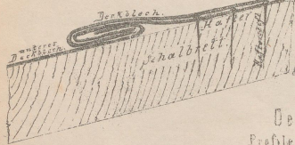
Liegender Falz in Naturgröße.
