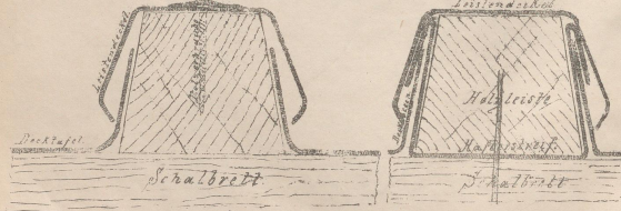
Deckleiste Profile in Naturgröße.
