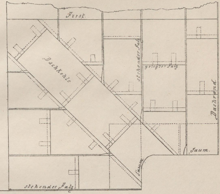
Giebelrandumbug.
