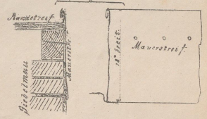
Eindeckung des Dachrandes Durchschnit
