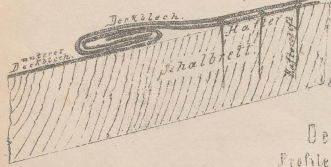
Liegender Falz in Naturgröße.
