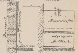
Eindeckung der Mauerviren Durchschnit
