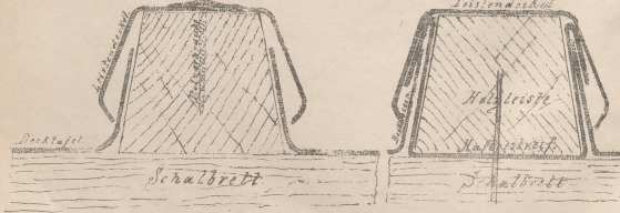
Deckleisten in Naturgröße.
