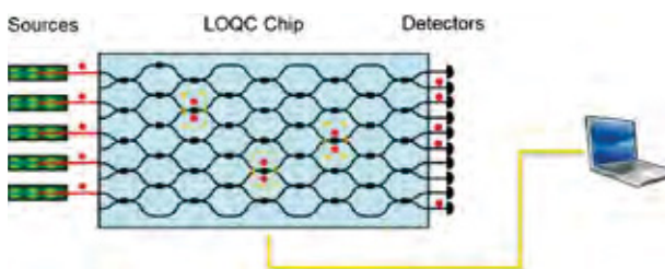
Vereinfachtes Blockschaltbild eines zukünftigen photonischen Quantencomputer auf Basis von photonischen integrierten Schaltungen. Simplified block diagram of a future photonic quantum computer using photonic integration.
