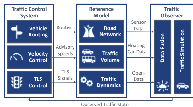
Systemstruktur des geschlossenen Regelkreises. System structure of the closed control loop.
