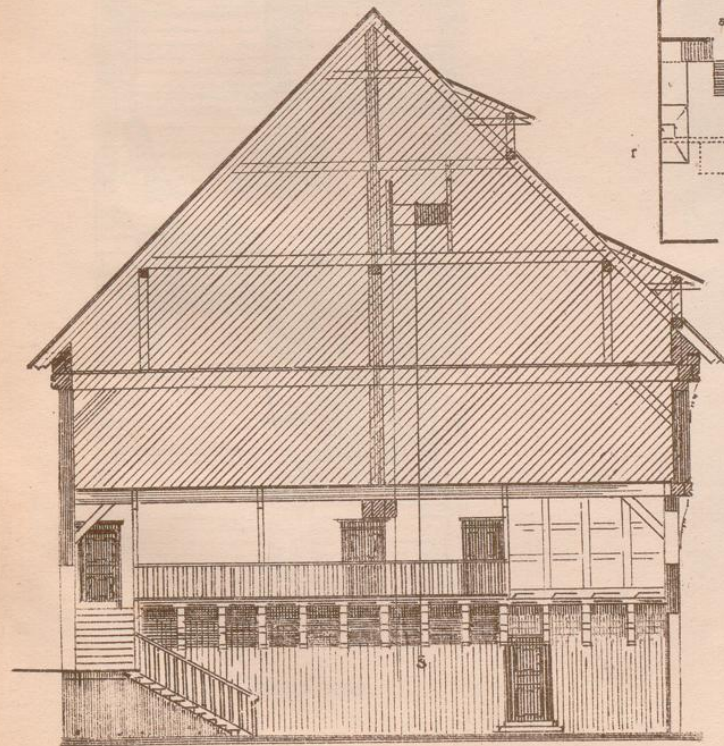
Querschnitt nach ab des Grundrisses.
