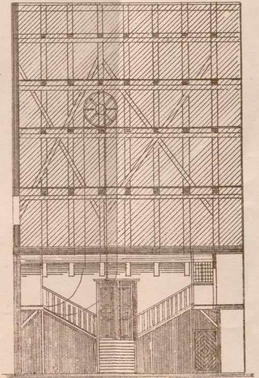
Längenschnitt nach rd des Grundrisses.
