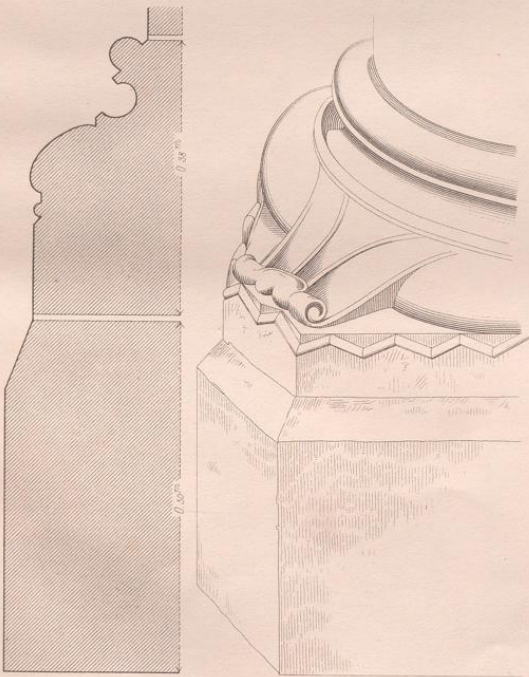
Fig. 16. Cathedrale zu Paris Ende d. XIII. Jahrh. n.V.I.D.
