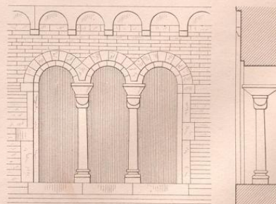
Fig 245. Gekuppelte Fenster Anf. XII. Jahrh. n. V. I. D.
