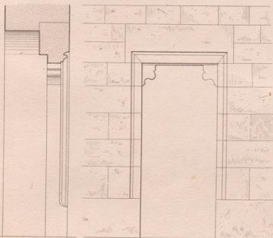
Fig. 313. Thüre vom Ende d. XIII. Jahrh. n.V.D.
