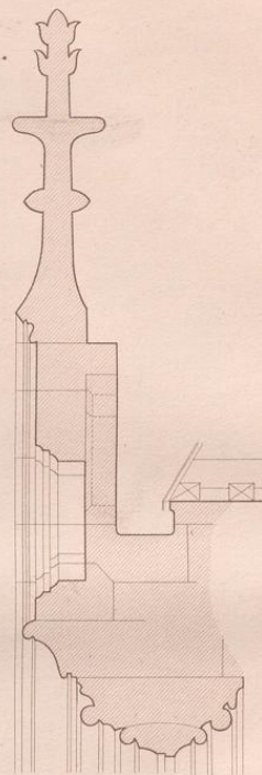
Schnitt durch die Giebelspitze.
