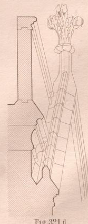
Schnitt nach e-f.
