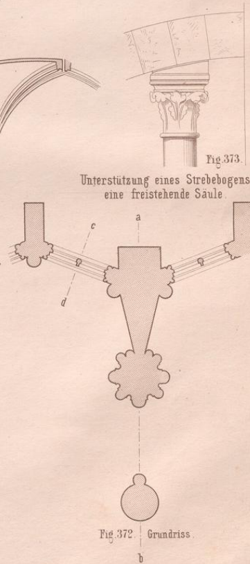
Strebesystem d. Cathedrale z. Chalons XIII. Jahrh. n. Ungew.
