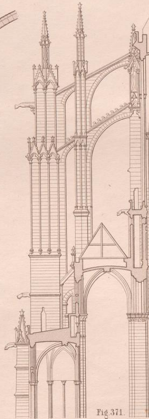
Schnitt nach c-d.
