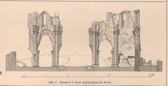
Abb. 5. Schnitt E-F durch das Querhaus der Kirche.
