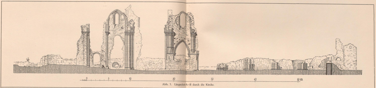
Abb. 3. Längsschnitt A-B durch die Kirche.
