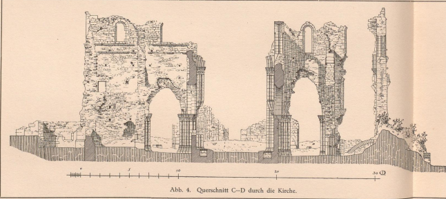
Abb. 4. Querschnitt C-D durch die Kirche.
