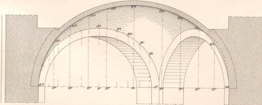
Schnitt E.G. Fig. 5.
