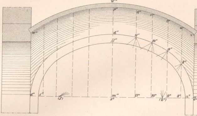
Schnitt A.B. Fig. 3.
