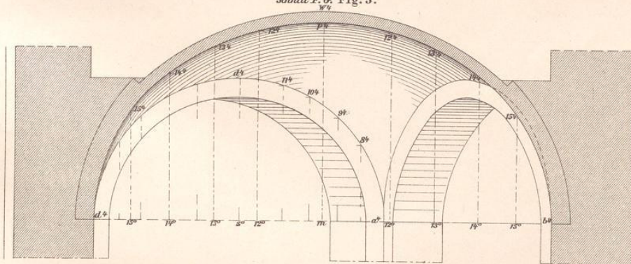
Schnitt E.G. Fig. 5.
