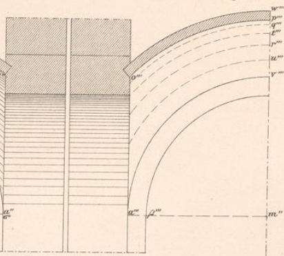
Schnitt C.D. Fig. 4.
