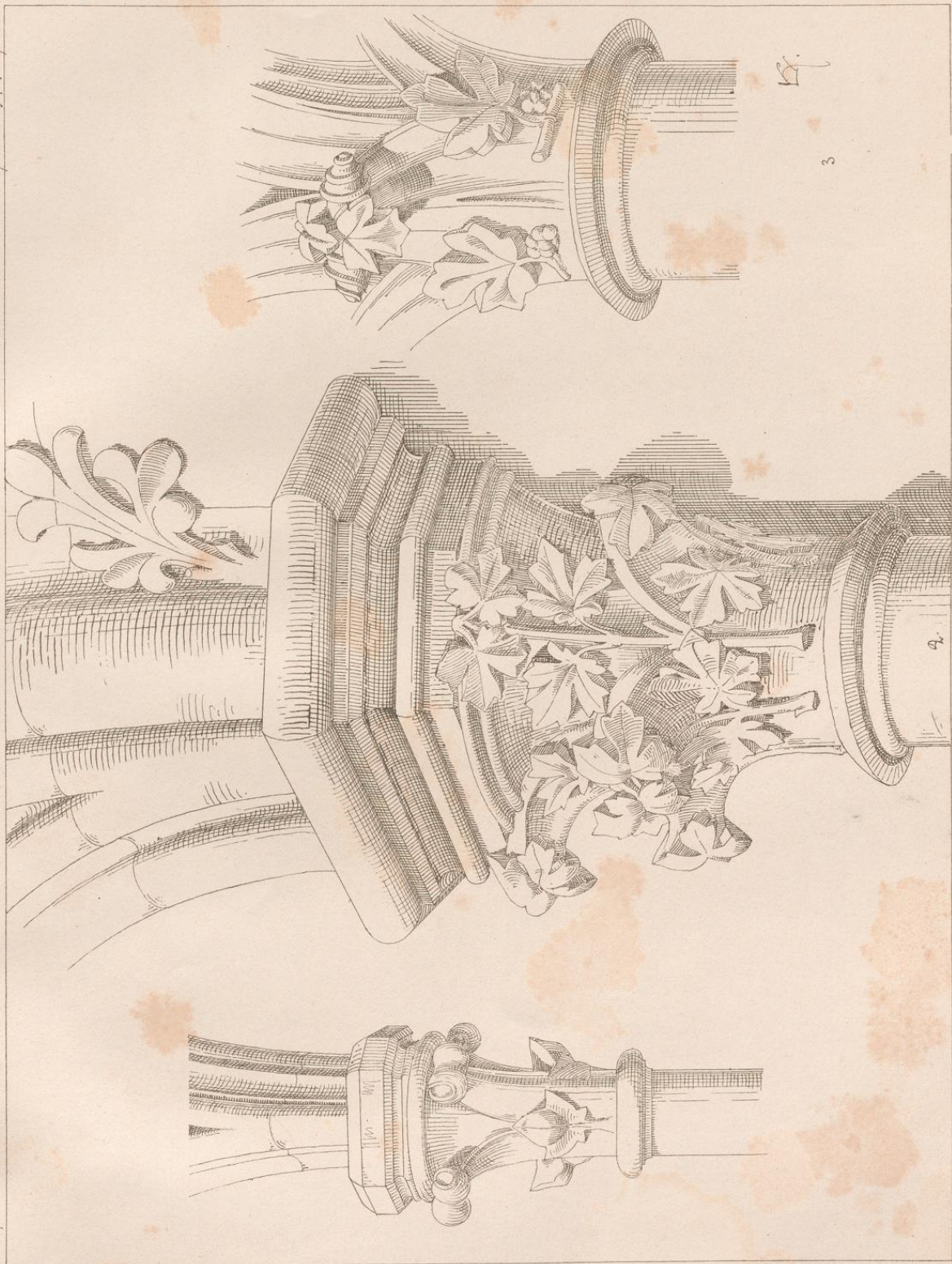
4. Kopfstück aus der St. Chapelle zu Paris. 2. Kopfstück von der Nord-Seite des Jumeau. 3. Kopfstück von der West-Seite.
