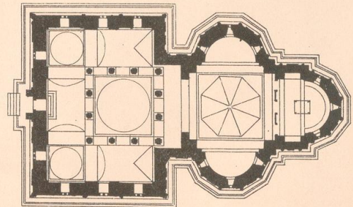
Fig. 20. Grundriss 1:300 der Biserica Curtea de Arges.
