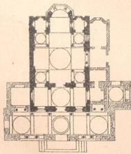
Fig. 12. Grundriss der Marienkirche (S. Theotokos) in Constantinopel.
