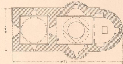
Fig. 26. Grundriss 1:200 der Kirche zu Petrouz.
