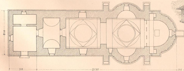
Fig. 29. Grundriss 1:200 der Kirche zu Burdaschény.
