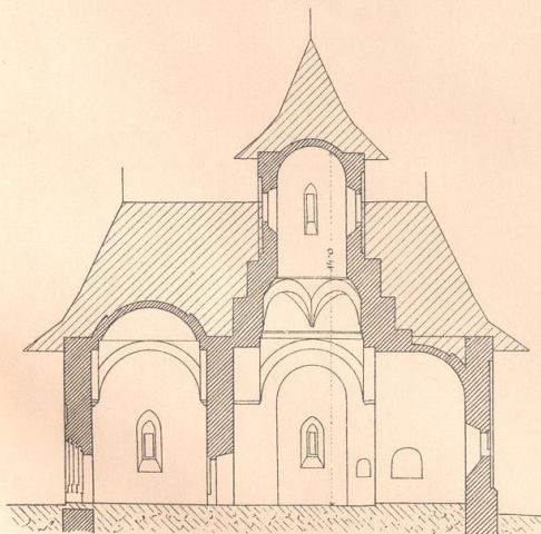
Fig. 27. Längenschnitt 1:200 der Kirche zu Petrouz.
