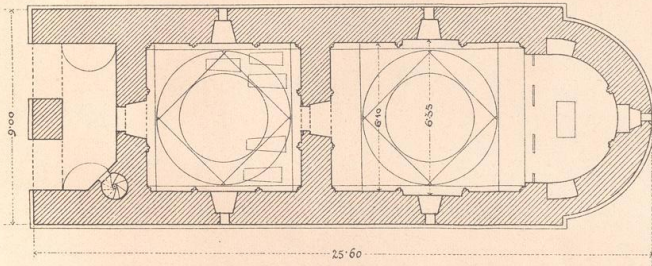
Fig. 35. Grundriss 1 : 200 der Kirche zu Parhautz.
