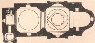
Fig. 30. Grundrisskizze der Spitalskirche zu Roman.
