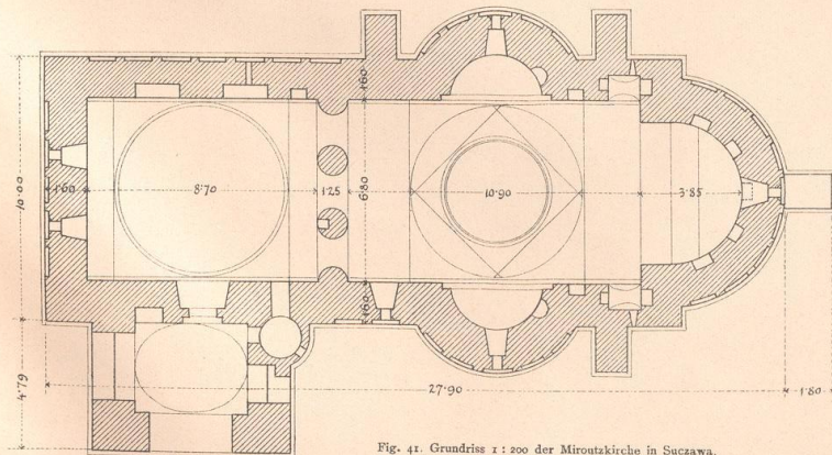
Fig. 41. Grundriss 1 : 200 der Miroutzkirche in Suczawa.
