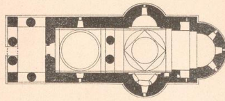
Fig. 31. Grundrisskizze der Kirche zu Alt-Itzkany.
