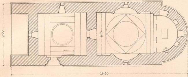
Fig. 33. Grundriss 1 : 200 der Kirche zu Reuseni.
