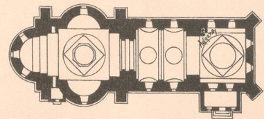
Fig. 50. Grundrisskizze der Episcopie in Roman.
