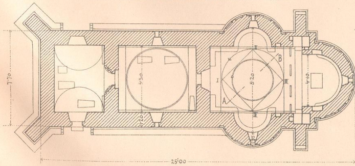
Fig. 48. Grundriss 1:200 der ehemaligen Klosterkirche in Woronez.
