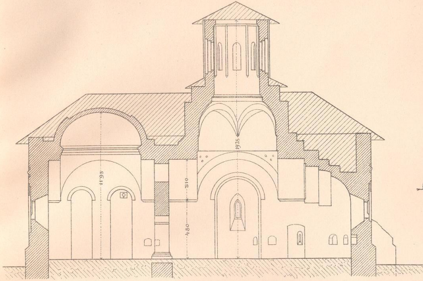
Fig. 42. Längenschnitt 1:200 der Miroutz-Kirche in Suczawa.
