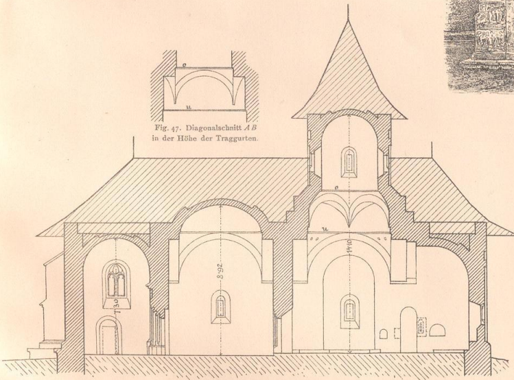
Fig. 46. Längenschnitt 1:200 der ehemaligen Klosterkirche in Woronez.
