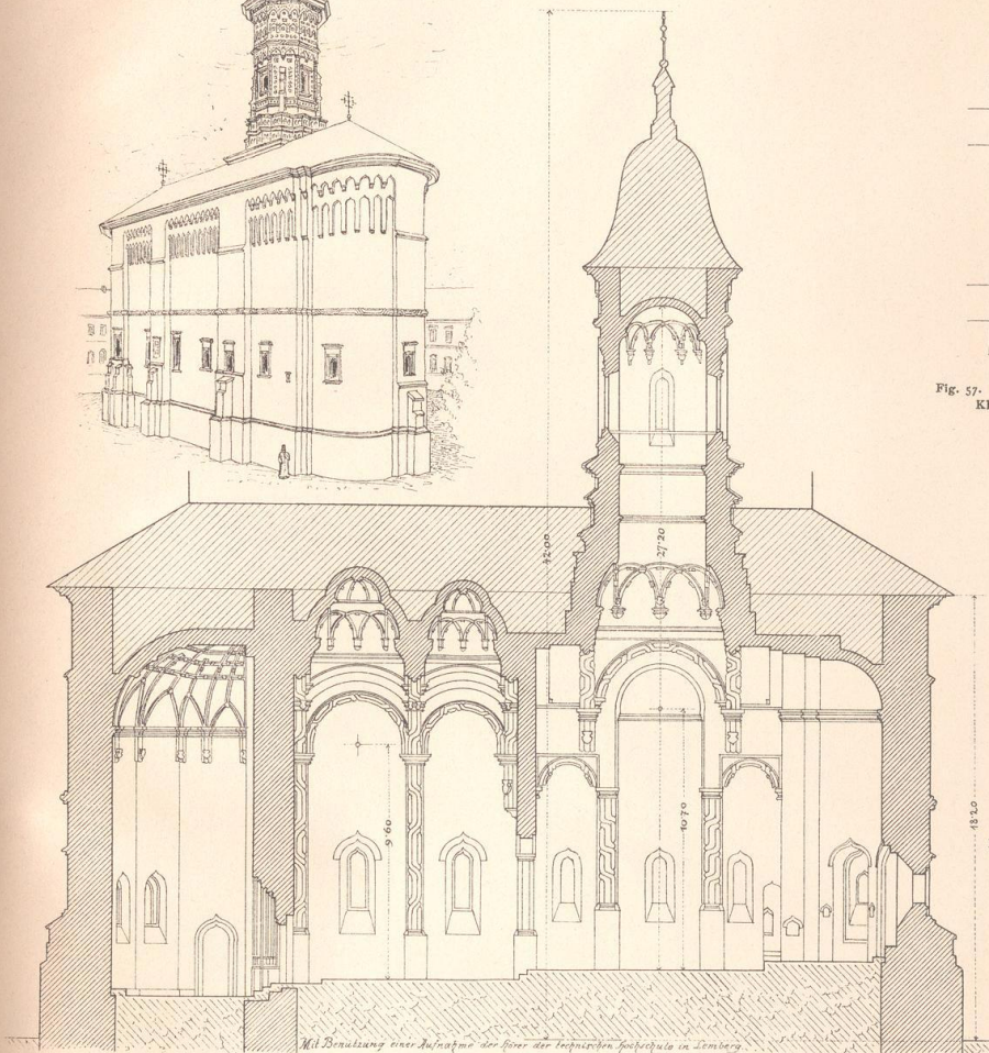
Fig. 52. Längenschnitt 1 : 200 der Klosterkirche zu Dragomirna.
