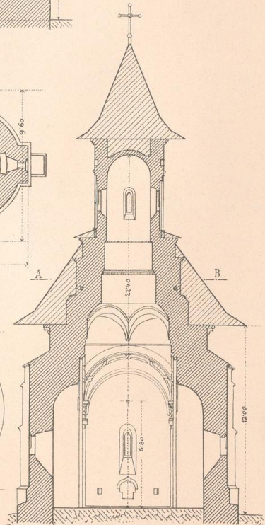
Fig. 55. Schnitt 1 : 200 der Kirche in Solka.
