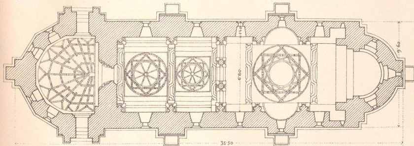
Fig. 53. Grundriss 1 : 200 der Klosterkirche zu Dragomirna.
