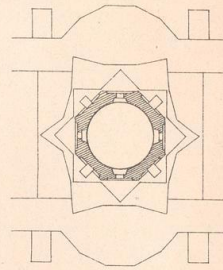
Fig. 57. Kuppel-Unterbau 1 : 200 der ehemaligen Klosterkirche zu Watra-Moldawitza.
