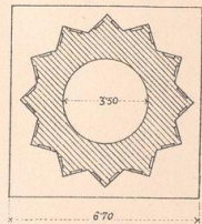
Fig. 56. Kuppel-Unterbau 1 : 200 der griech.-orient. Kirche zu Solka.
