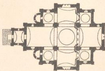
Fig. 148. Sretenskaja-Kirche in Odessa.
