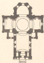
Fig. 151 u. 152. Griech.-orthodoxe Kirche in Odessa.
