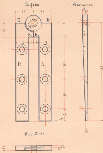
2 Stück Charniertheile A und B (1 Stück rechts, 1 Stück links)
