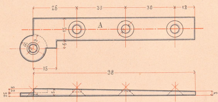
2 Stück Charniertheile A und B (1 Stück rechts, 1 Stück links)
