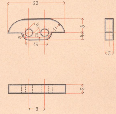
1 Stück Anschlag B.
