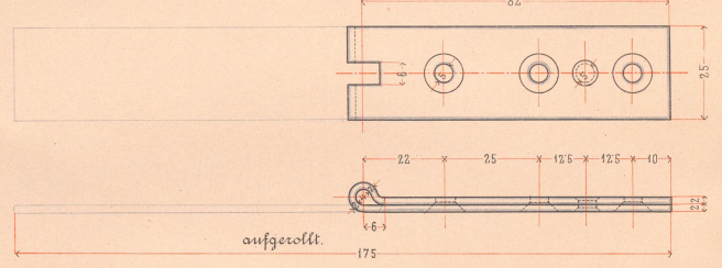
2 Stück Charnierbänder A
