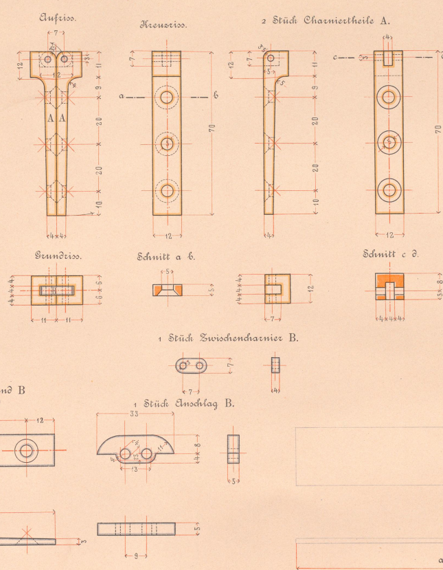
2 Stück Charnierbänder A
