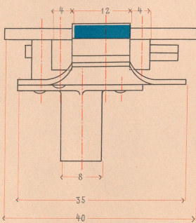
Seitensicht, Ansicht und Schnitt: h i k l.
