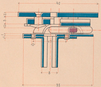
Seitensicht, Ansicht und Schnitt: h i k l.
