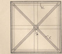
GRUNDRISS DES LEHRGERÜSTES
