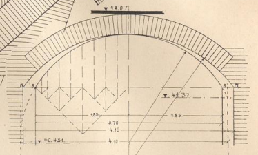
BOGEN-F. UND KONSTRUKTION DER VERSCHIEDENEN ANSCHNITZPUNKTE.
