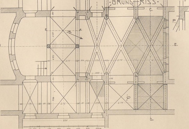
MASSTAB FÜR DEN GRUNDRISS. SCRIBA, MODERNE DECKEN UND GEWÖLBE
