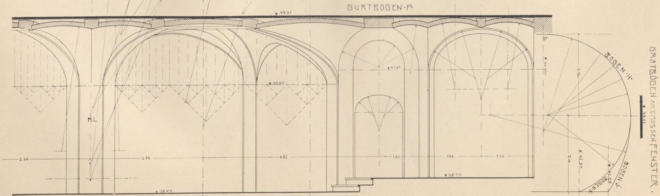
OFFENES KLOSTERGEWÖLBE MIT STICKKAPPEN.
