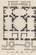
4. Villa zu Chiswick. Von Inigo Jones.
