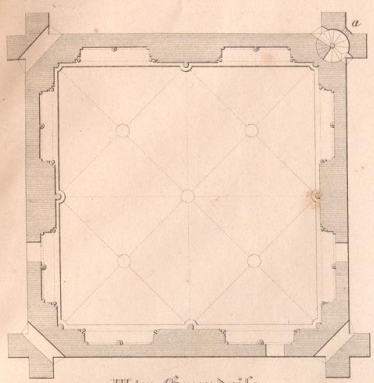
IIIter Grundriß.
