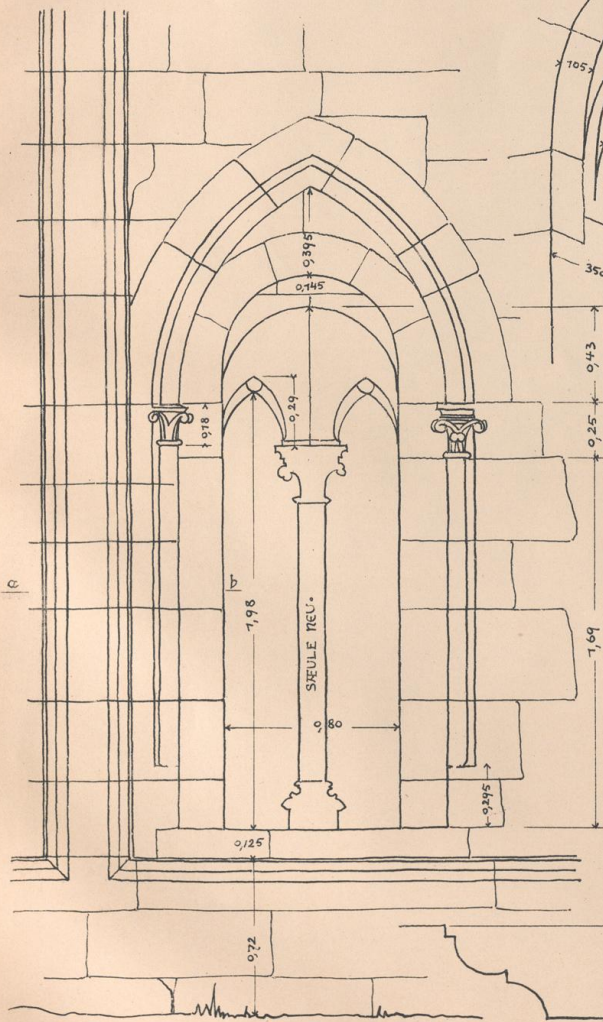
VORHALLE RECHTS VOM PORTAL 1:20
