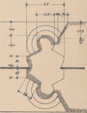
PFOSTEN UND GEWÄNDE 1:10
