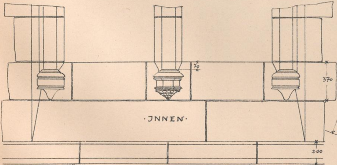
• S-ELISABETHKIRCHE • • UNTERE FENSTER IM LANGSCHIFF • 1:20
