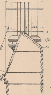
PFOSTEN UND GEWÄNDE 1:10
