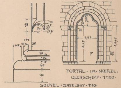
SOCKEL · DASELBST · 1:10.
