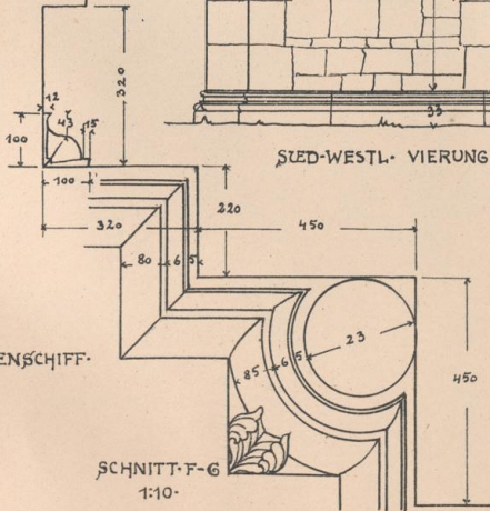
PROFIL-D · 1:10.
