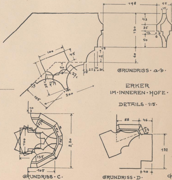
GRUNDRISS • d
