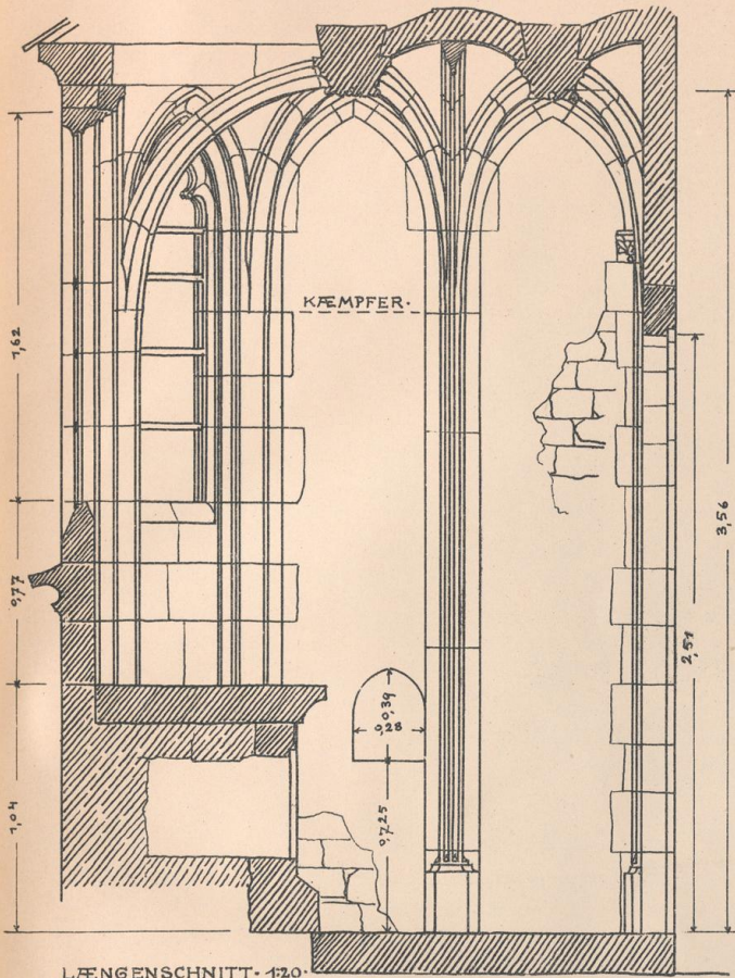
LÄNGENSCHNITT • 1:20
