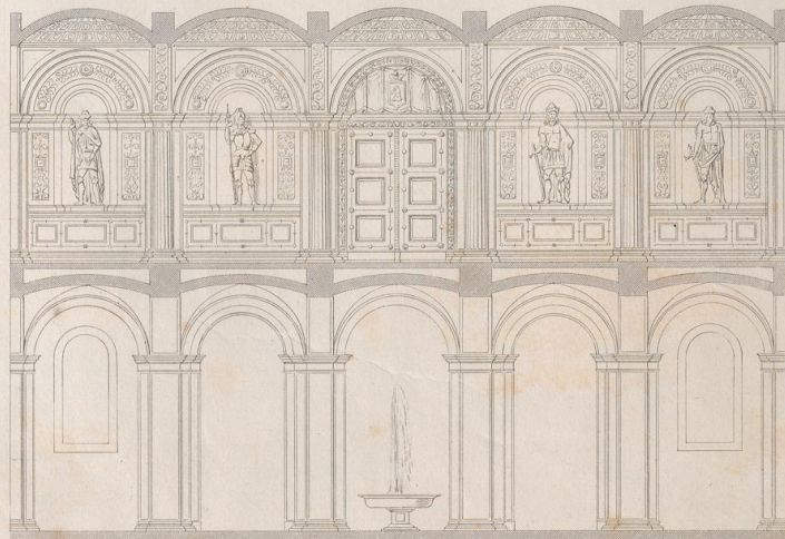
DURCHSCHNITT DURCH DAS VESTIBÜLE U. DEN DARÜBERLIEGENDEN GROSSEN VERSAMMLUNGSAL NACH DOPPELTEM MAASSTABE.
