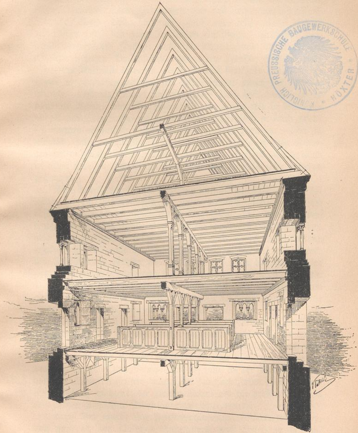
Tunenperspektive des Rathauses.
