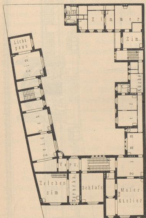
II. Obergeschoss 60 .
